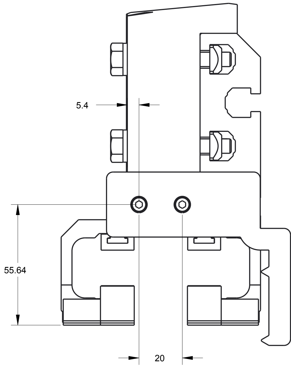
DETAIL A SCALE: 1/1
