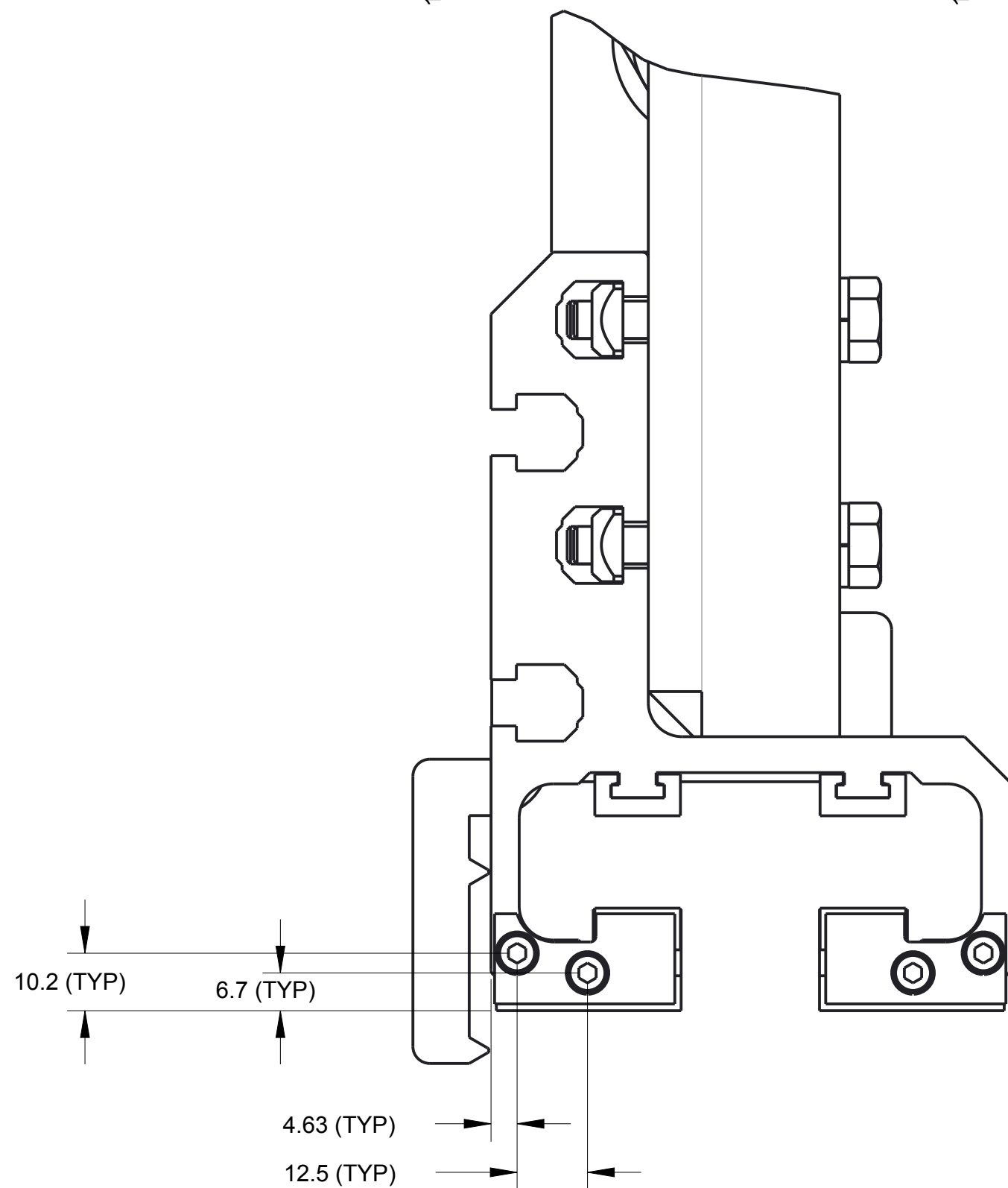
DETAIL B SCALE: 1/1
